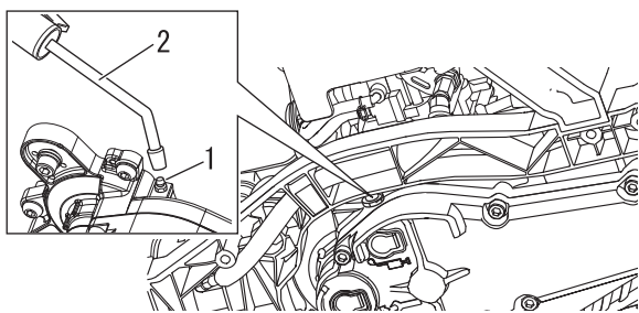
1. Smeernippel
