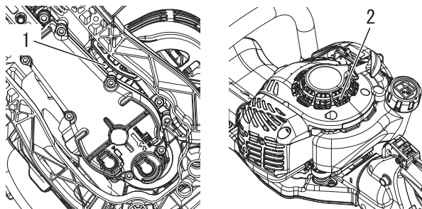
1. Koelribben van de cilinder 2. Koelluchtinlaat
